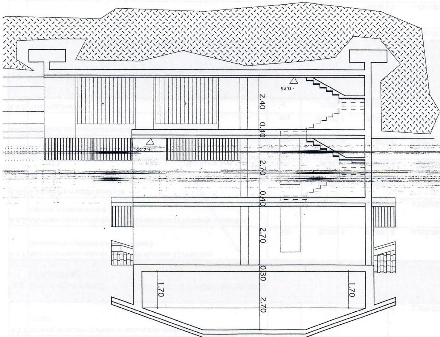
SEZIONE B.B IN VARIANTE Scala 1/100
